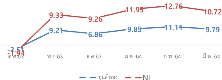
NWC/NI
